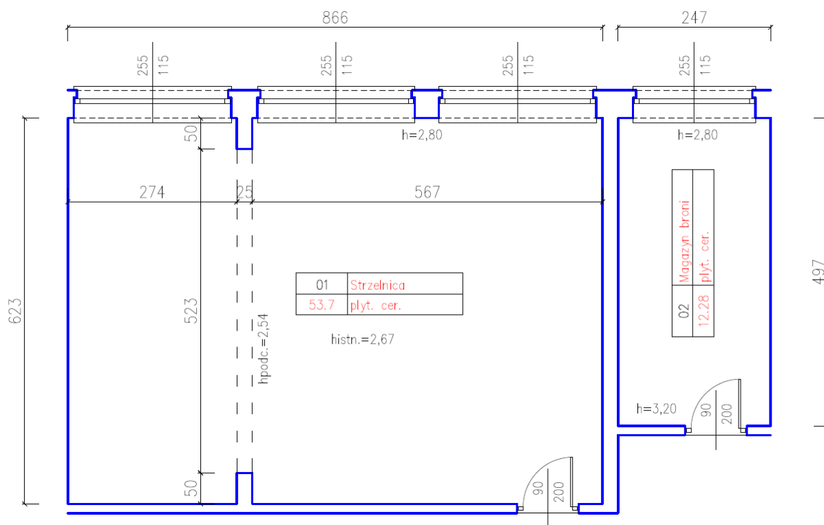
Rys. nr 1 – rzut pomieszczeń
